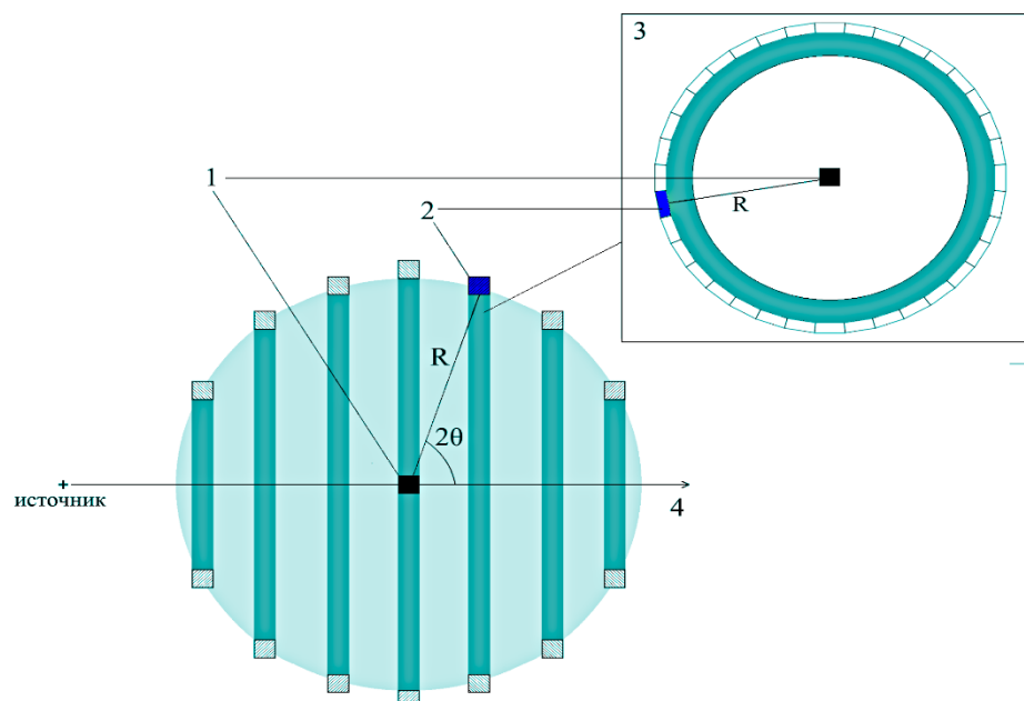
Рисунок 1.1.10.4 — Конфигурация детектора “СФЕРА”, синим цветом выделен счетчик, рассматриваемый в модели: 1 - образец, 2 - нейтронный счетчик, 3 - кольцевой детектор
