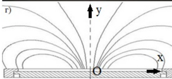
Рис. 1.1.2.1. Связь формы эрозии мишени магнетрона с свечением плазмы и конфигурацией магнитного поля
