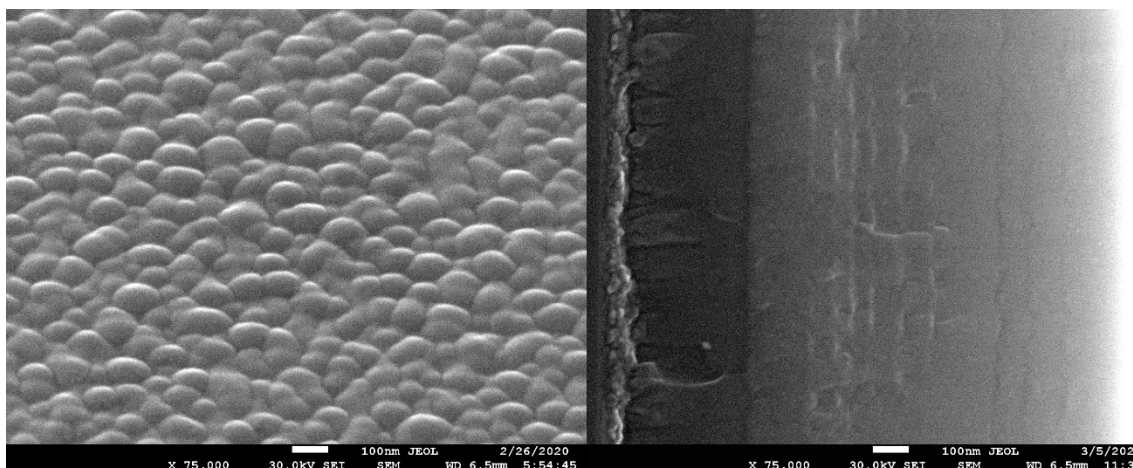
Рис. 1.1.1.6. Микрофотографии плёнки образца №1, осаждённой при 200°С, давлении Ar 1,4 мТорр.
